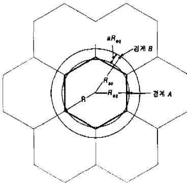
그림 1. 소프트 핸드오프 경계
