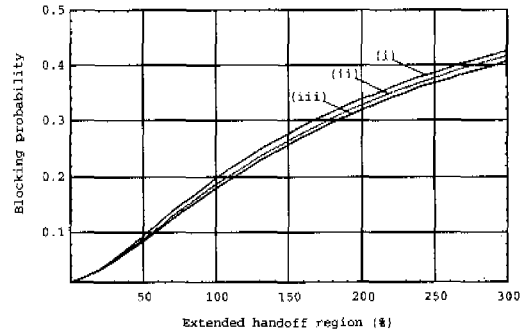
그림 5. 이동국 속도와 소프트 핸드오프 영역 변화가 블록킹율에 미치는 영향 (i) V_{max}=10 Km/hr (ii) V_{max}=60 Km/hr (iii) V_{max}=120 Km/hr
