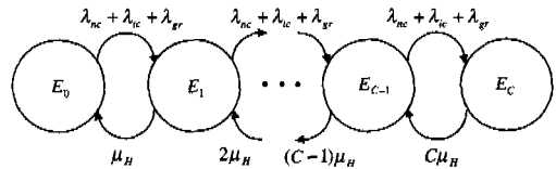
그림 3. 상태전이도
