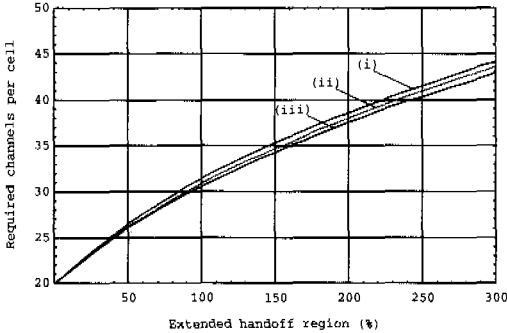
그림 6. 소프트 핸드오프 영역 증가시 P_B=0.01 유지에 필요한 채널 수
