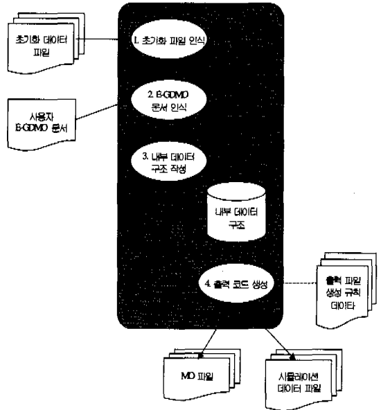
그림 17. 확장된 GDMO 컴파일러의 수행과정
