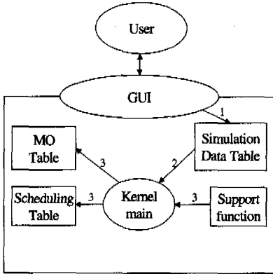
그림 9. GUI를 통한 SDT 초기화 및 동작
