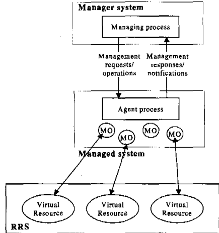
그림 2. 관리자, 에이전트, 그리고 RRS와의 관계
