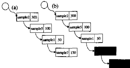
그림 5. 스케줄링 테이블 예
