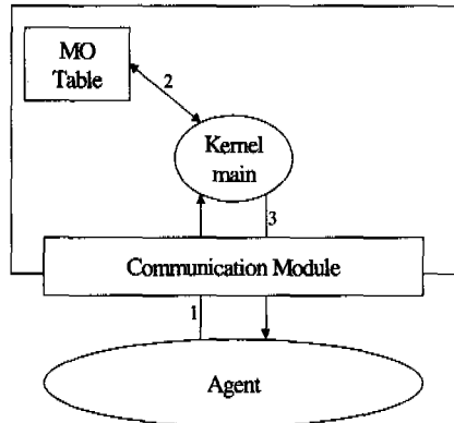
그림 10. 에이전트로부터 요청된 속성의 처리 과정
