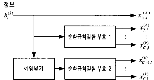
그림 2. 터보 부호기
