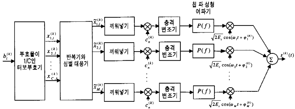
그림 1. 송신기
