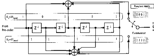
그림 3. Punctured 2진 길쌈 부호기.
