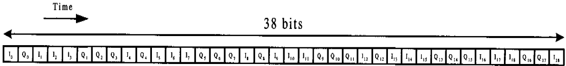
그림 6. TC 256-QAM 변조기 입력 trellis 그룹.
