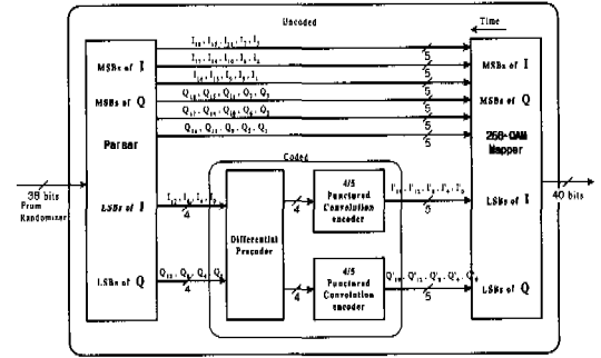
그림 5. TC 256-QAM 변조기.
