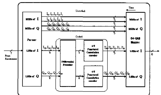
그림 2. TC(Trellis Coded) 64-QAM 변조기.
