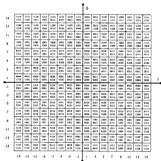
그림 8. 256-QAM 성좌도.
