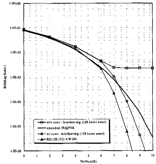
그림 11. 128 심볼 burst error에 대한 BER 성능.
