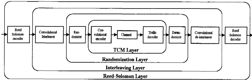
그림 1. FEC의 구조
