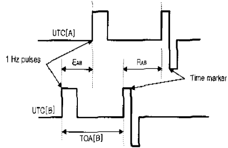
그림 6. TDF2에 적용된 시각전송 원리
