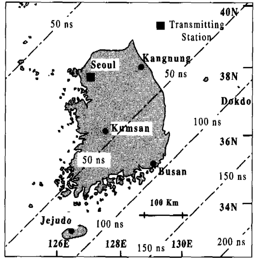
그림 4. 송신지구국(서울)~수신지구국간 거리에 따른 차동보정 방식의 시각 error contour(3축에 대한 예측 오차가 각각 2 km인 경우)
