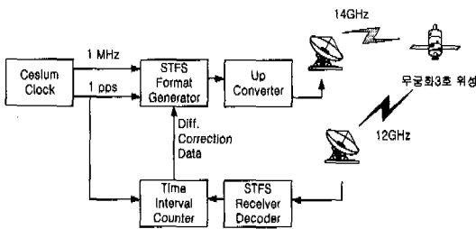
그림 3. 차동보정 방식을 적용한 송신기준국의 동작구성도
