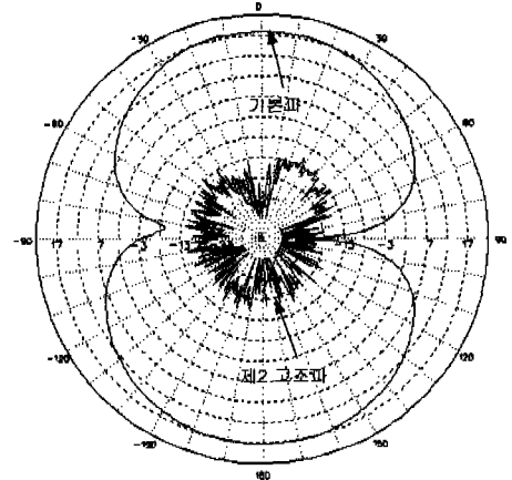
(c) E-plane 방사패턴 (기본파 및 제2고조파)
