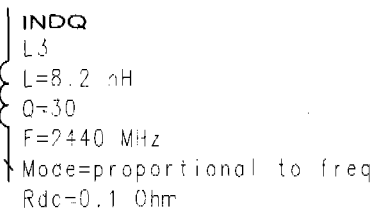
(b) 칩인덕터 등가모델
