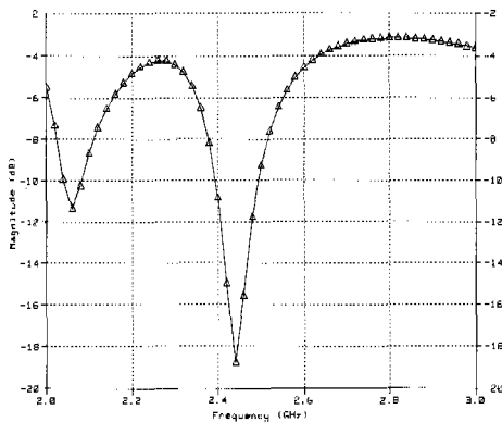
그림 9. 안테나 반사손실 (시뮬레이션)
