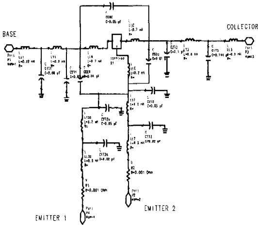
그림 3. HBBF-0450 BJT 패키지 기생성분 모델링
