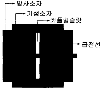
(a) 설계된 단일 방사소자의 구조
