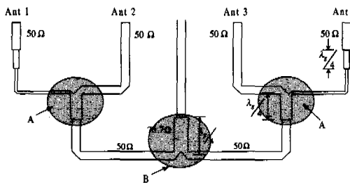
그림 4. 1 \times 4 배열안테나의 급전 네트워크 구조
