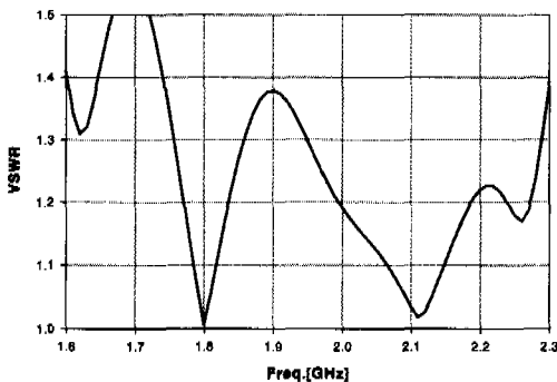
그림 7. 1×4 배열안테나의 VSWR 특성
