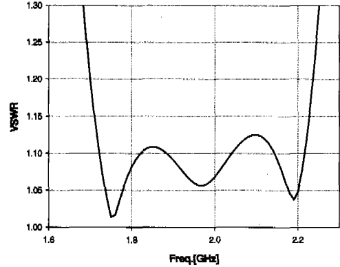
그림 3. 단일 방사소자의 VSWR 특성
