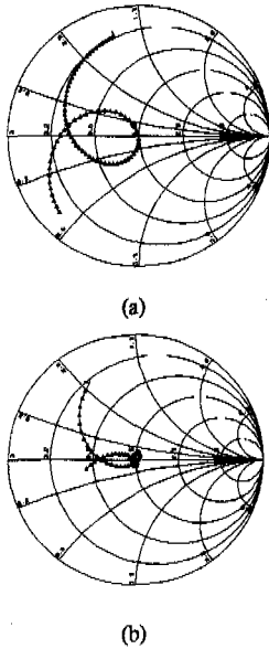
그림 2. 단일방사소자의 임피던스 특성 (a) 기생소자를 사용하지 않은 경우 (b) 기생소자를 사용한 경우
