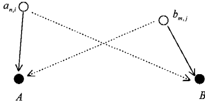
(a) BS←MS 간섭 (A: 역방향 링크, B: 역방향 링크)
