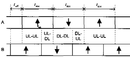
(c) 동기가 일치하지 않은 경우
