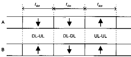
(b) 서로 다른 프레임 구조를 갖고 동기가 일치한 경우
