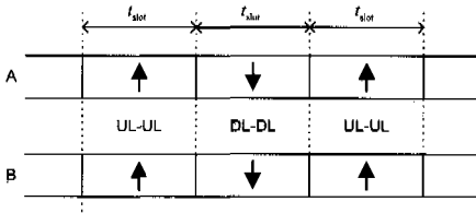
(a) 동일한 프레임 구조를 갖고 동기가 일치한 경우
