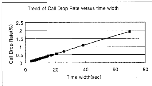
그림 7. 시간폭에 따른 호 절단율 추정
