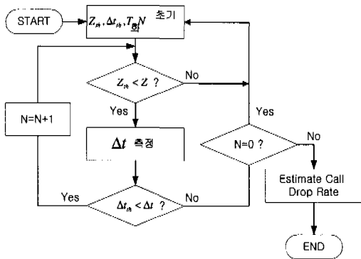
그림 3. 호 절단 추정 알고리즘
