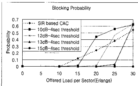
그림 11. 각 전력레벨 4sec 한계치를 기준으로 한 경우와 SIR을 근거로 한 CAC인 경우 호 거부율 비교
