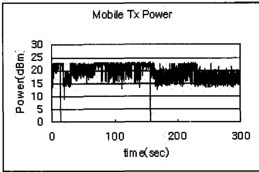
그림 6. 시간에 따른 단말기 전송 전력
