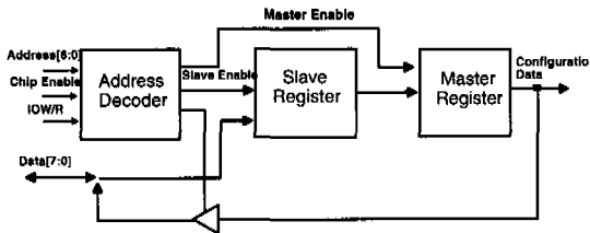
그림 7. 마이크로프로세서 접속부
