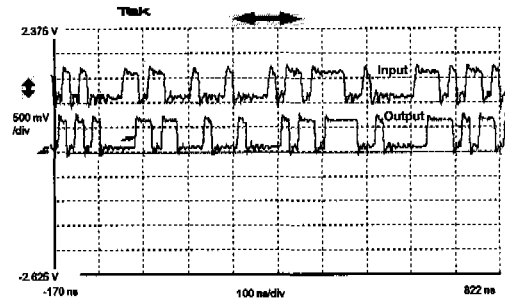
그림 10. 스위치 소자의 측정된 입출력 파형
