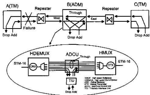
그림 1. 선형 전송망
