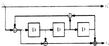
그림 2.1 재귀 조직 길쌈 부호(rate 1/2, 8state)
