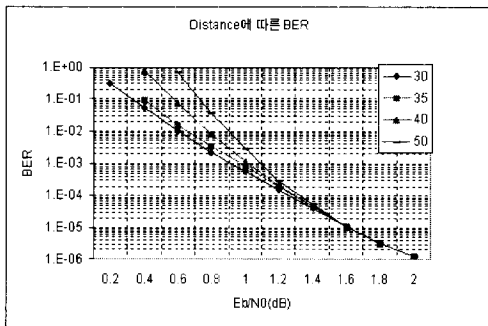
그림4.1 distance에 따른 BER
