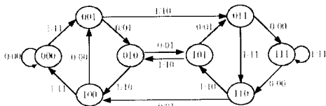
그림 2.2 상태도
