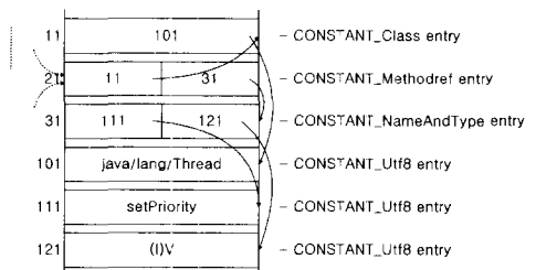
(a) Thread.setPriority(I)V에 의한 수정
