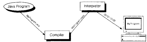
그림 1. 자바 프로그램의 수행과정 Fig. 1 Execution Process of Java Program
