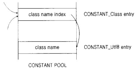
그림 7. 상수 풀 내에 두 개의 요소를 갖는 클래스
