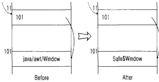
그림 8. 클래스 레벨의 수정
