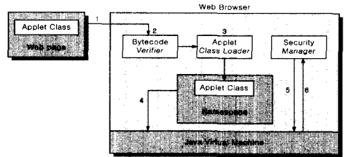
그림 5. 자바 애플릿의 보안 처리 과정 Fig.5 Security Management Process of Java Applet
