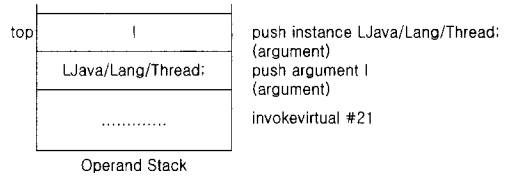
그림 10. 메소드 호출 명령을 위한 Operand 스택과 명령어 순서
