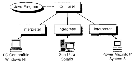
그림 2. "Write Once, Run Anywhere"를 보여주는 Java 수행 모델
