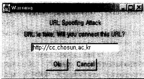
그림 16. URL 위장 공격에 대한 경고창 Fig. 16 Warring Windows for URL Spooltion Attack
