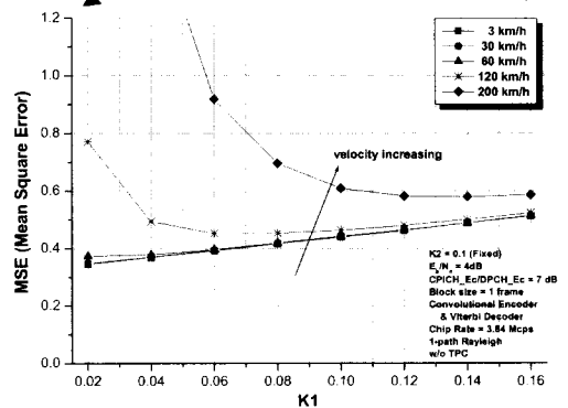
(b) 필터 계수 K1 의 값이 좁은 범위일 때
