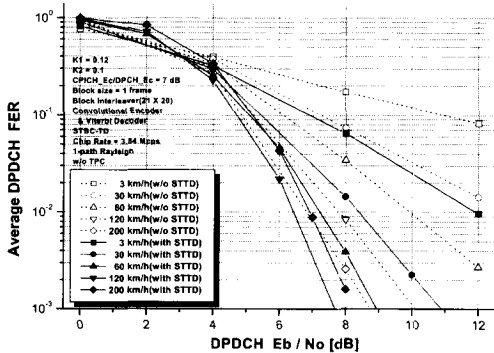
그림 13. IIR 필터 구조에서 이동국의 속도와 E_b/N_0 에 따른 FER
