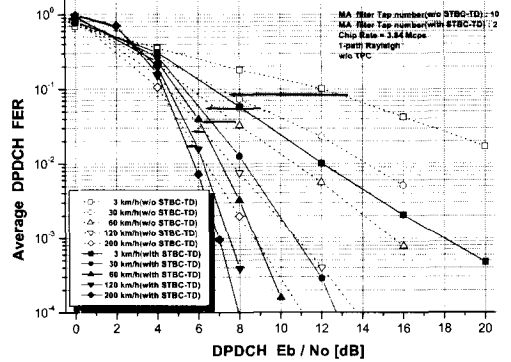
그림 9. 이동 평균 필터 구조에서 이동국의 속도와 E_b/N_0 에 따른 FER
