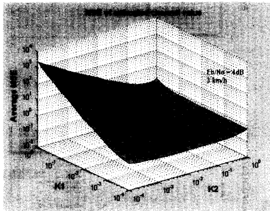
그림 11 (a). IIR 필터 계수 K1 과 K2 에 따른 채널 추정 값의 MSE ( E_b/N_0=4\text{dB} , 3\text{km/h} )
