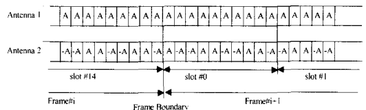
그림 2. 송신 다이버시티 환경에서의 CPICH 변조 패턴
