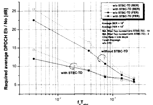
그림 10. 이동 평균 필터 구조에서 최대 도플러 주파수에 대해 평균 BER 10^{-3} , 평균 FER 10^{-2} 을 얻기 위해 요구되는 E_b/N_0
