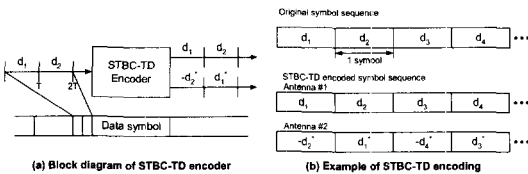
그림 3. STBC-TD 부호화기
