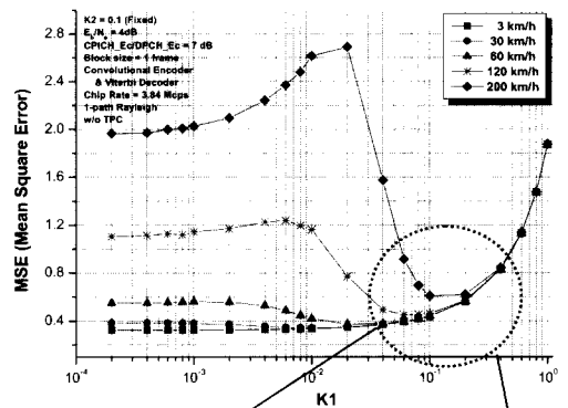
(a) 필터 계수 K1 의 값이 넓은 범위일 때
