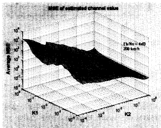
그림 11 (b). IIR 필터 계수 K1 과 K2 에 따른 채널 추정 값의 MSE ( E_b/N_0=4\text{dB} , 200\text{km/h} )
