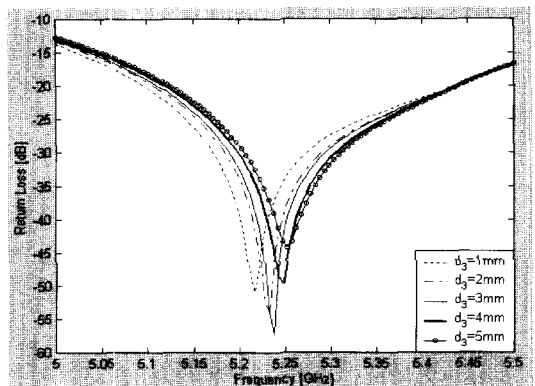
그림 14. 역 U-슬롯 모양 간격 d_3 변화에 따른 반사계수
