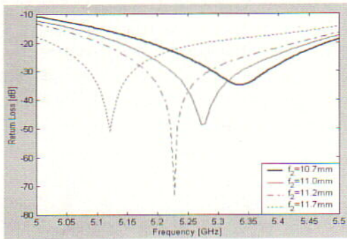
그림 15. 동축 급전의 위치 f_2 변화에 따른 반사계수
