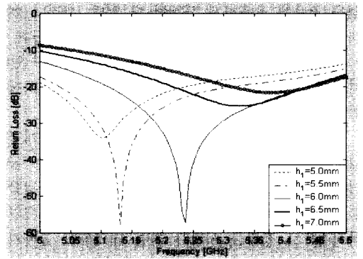
그림 9. 큰 U-슬롯 모양 위치 h_1 변화에 따른 반사계수
