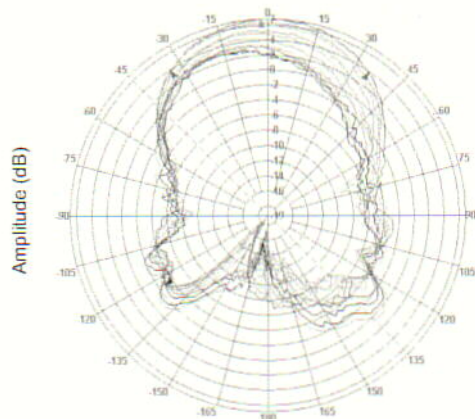
(b) H-평면
