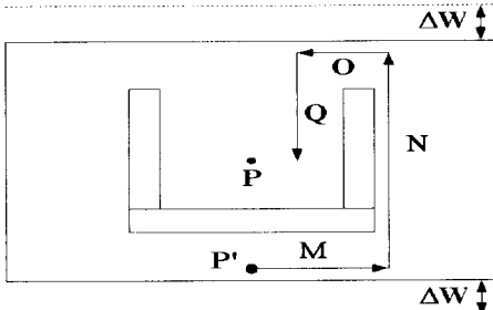
그림 4. 두 번째 공진을 일으키는 전류통로길이
