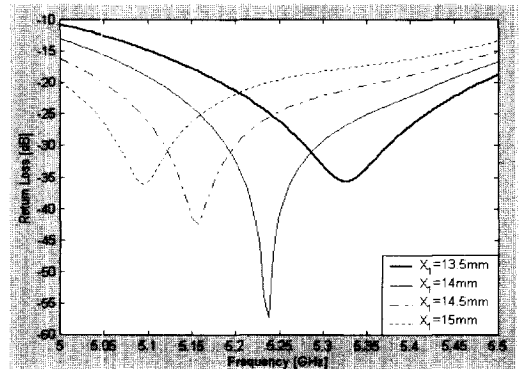
그림 6. 큰 U-슬롯 모양 가로길이 X_1 변화에 따른 반사계수
