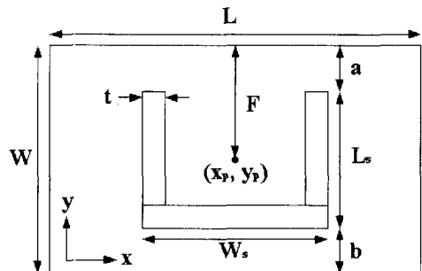
그림 2. U-슬롯 안테나
