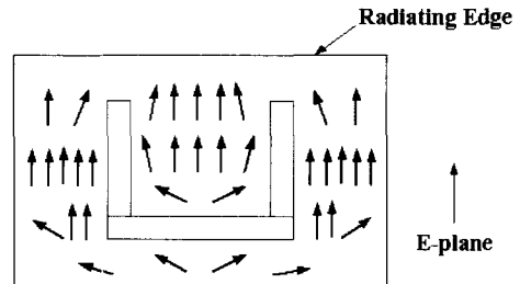
그림 1. U-슬롯에 의해 교란된 전류분포
