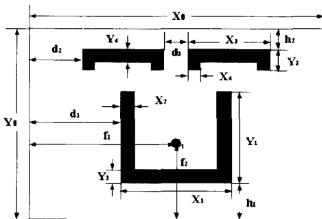
그림 5(a). 설계된 안테나 구조
