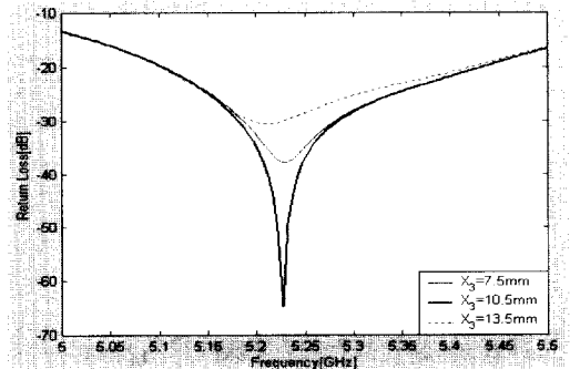
그림 10. 역 U-슬롯 모양의 가로길이 X_3 변화에 따른 반사계수
