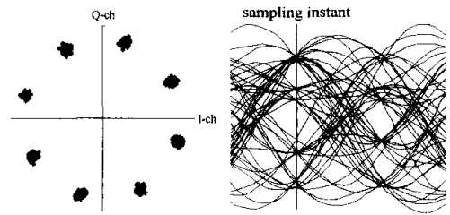
(b)8PSK (α=0.3, IBO=5dB)
