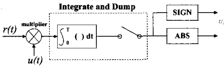
그림 15. 준최적 상관수신기의 동작 구성도
