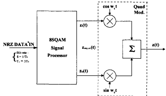
그림 4. 8SQAM 변조기의 동작구성도
