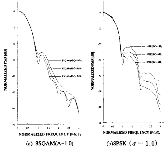
그림 10. 비선형채널 환경에서 IBO에 따른 8SQAM과 8PSK 신호의 전력 스펙트럼 밀도
