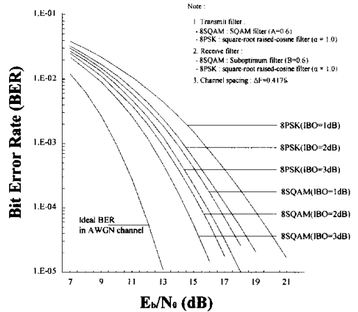
그림 17. 비선형 증폭 다중채널 간섭 환경 (SCPC-FDMA)에서 HPA의 IBO에 따른 8SQAM과 8PSK의 수신 BER 성능 ( \Delta F = 0.417f_b )
