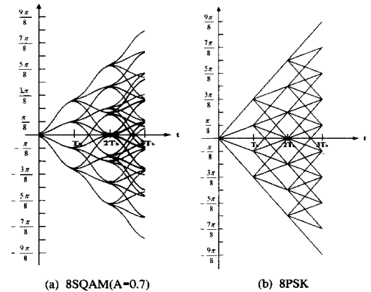
그림 8. 8SQAM과 8PSK 신호의 위상 천이도
