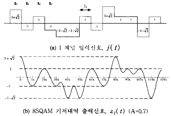
그림 7. 8SQAM 출력신호 파형 (Note: T_s = 3T_b : 심볼 간격, T_b : 비트 간격)
