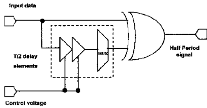
그림 3 HPSG의 회로도
