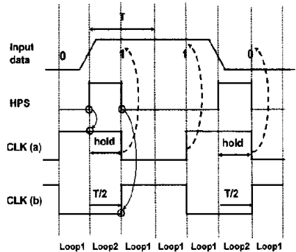
그림 6 MO의 타이밍도
