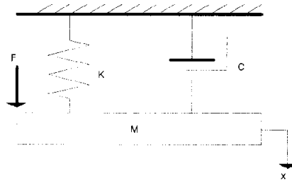
그림 3. 동적 시스템 모델의 구성
