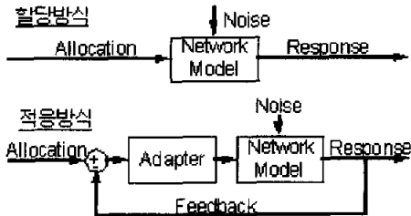
그림 1. 할당방식과 적응방식의 구조
