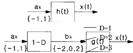
그림 1. 자기 기록 시스템 채널 모델
