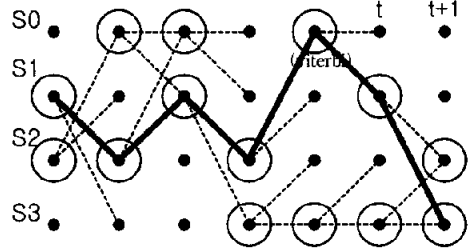
그림 4. M-알고리즘의 복호 트랜리스 예
