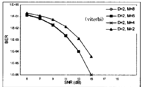
그림 6. EPR-4, D=2일 때 M의 변화에 따른 BER
