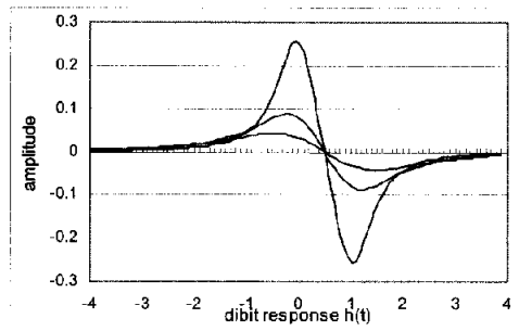
그림 3. D의 증가에 따른 이중 비트 응답
