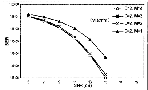
그림 5. PR-4, D=2일 때 M의 변화에 따른 BER
