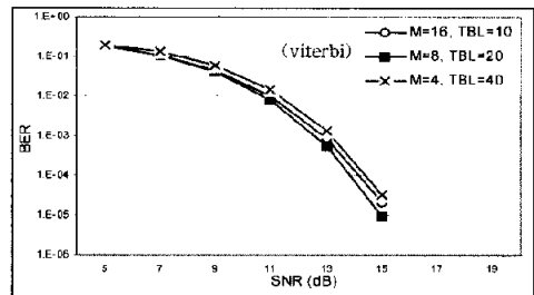
그림 9. EEEPR4, D2에서 같은 메모리 양을 사용할 때 성능차이 BER
