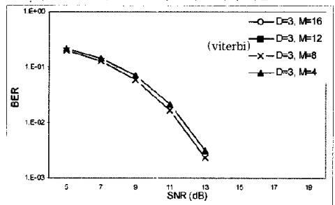
그림 7. EEPR-4, D=3일 때 M의 변화에 따른 BER
