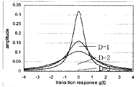
그림 2. D의 증가에 따른 고립 펄스 응답
