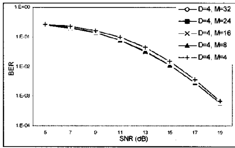
그림 8. EEEPR-4, D=4일 때 M의 변화에 따른 BER
