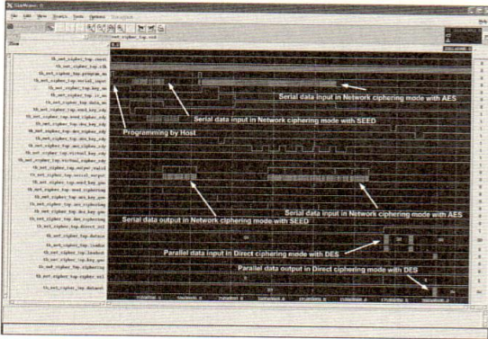
그림 10. 네트워크 암호모드의 전체적 시뮬레이션 결과 Fig. 10. Global simulation result in network ciphering mode
