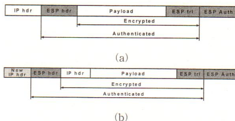
그림 1. IPsec의 ESP 모드에서 암호화 대상 (a)전송모드 (b)터널모드 Fig. 1. Encryption item in ESP mode of IPsec (a)transport mode (b)tunnel mode
