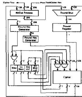
그림 4. AES의 H/W 구조 Fig.4. H/W structure of AES cryptosystem
