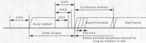
그림 2 IEEE 802.11 기본 액세스 방법
