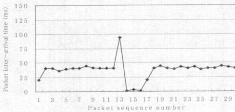
그림 15 DS 대역폭이 10 Mbps인 경우 프레임의 inter-arrival 시간
