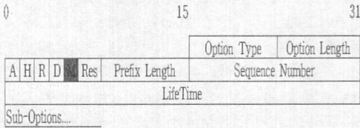
Fig 3. BU 메시지 형식
