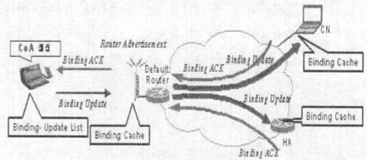
Fig 1. 이동 IPv6의 동작
