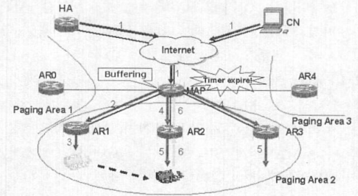
Fig 8. HMIPv6의 페이징 과정
