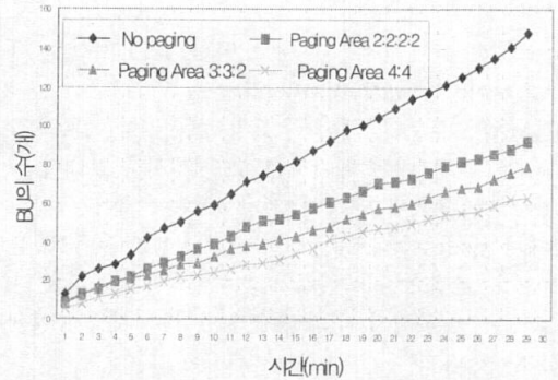
Fig 13. 페이징 영역 크기에 따른 누적된 BU의 수
