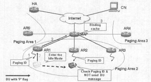
Fig 7. 페이징이 적용된 HMIPv6에서의 페이징 등록
