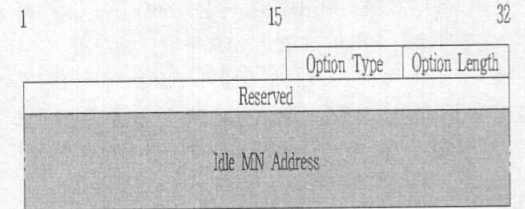
Fig 9. 페이징 요청 메시지의 형식
