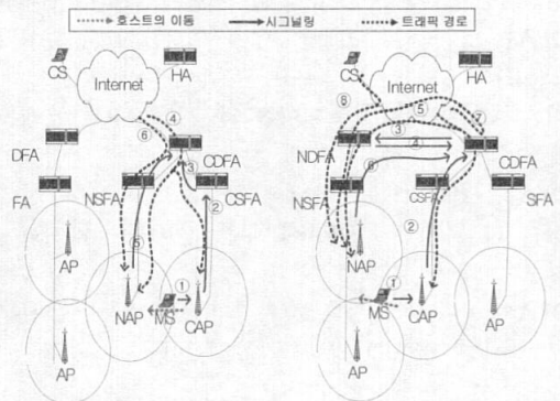
(a) 도메인 내 이동 (b) 도메인 간 이동 그림 3. CCFH 알고리즘을 적용한 시나리오 Fig. 3. Scenario for CCFH algorithm. (a)intra domain, (b)inter domain handoff.
