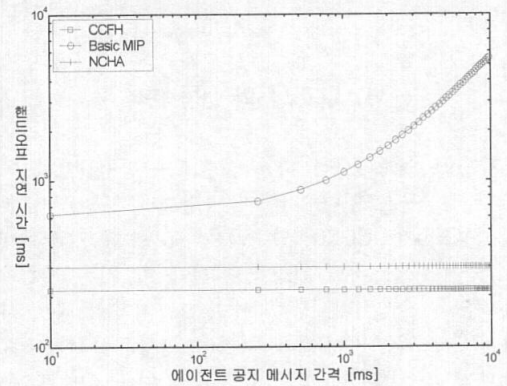
그림 5. 에이전트 공지 메시지 간격에 따른 각 알고리즘의 핸드오프 지연시간. (가정 : T_S \approx 200 ms, T_I \approx 70 ms, T_R \approx 20 ms, T_G \approx 400 ms, T_W = \text{Agent Advertisement interval}/2 ) Fig. 5. Handoff latency of each algorithm according to agent advertisement message interval.
