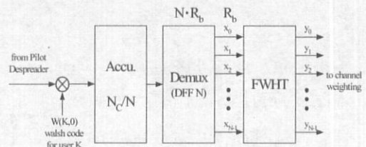
그림 2. 공유 accumulator를 이용한 제안된 구조
