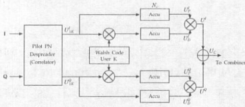
그림 1. 단일 채널의 기존 데이터 상관기
