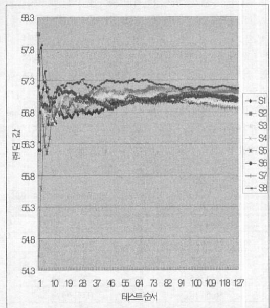
그림 3. 각 S박스에 대한 랜덤성 비교
