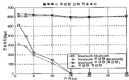
그림 9 블루투스와 무선 LAN간의 전송속도 측정
