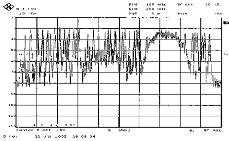
그림 2 블루투스 및 무선랜이 동작하는 스펙트럼
