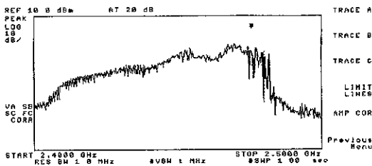
그림 8 무선랜과 셀룰라 폰의 전력스펙트럼
