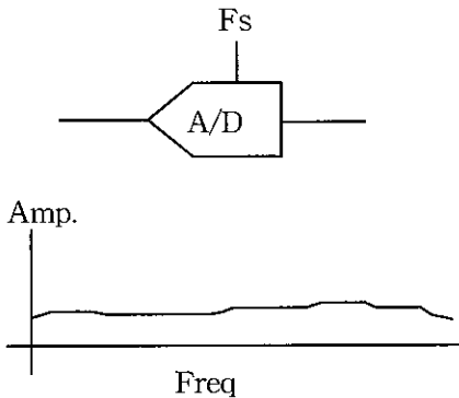
그림 2 2 (b) Noise Shaping Filter를 가진 A/D 변환기
