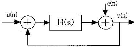
그림 2.7 Discrete-time 선형 Sigma-delta modulator 모델
