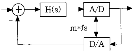
그림 2 3 Sigma-delta modulator 의 기본구성
