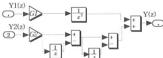
그림 4.3 디지털 오차 제거 로직
