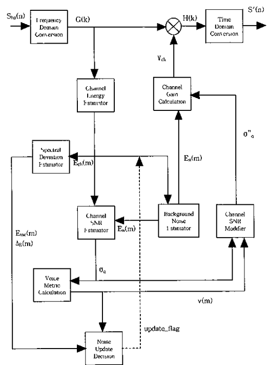
그림 1 EVRC의 잡음 억제 블록도
