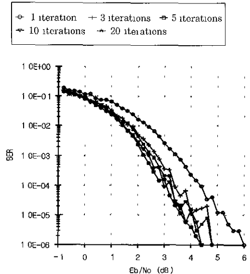
그림 9 디코딩 반복횟수에 따른 제안 코드의 성능
