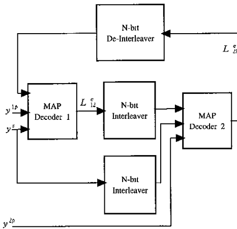
(b) Turbo 디코더 블록도
