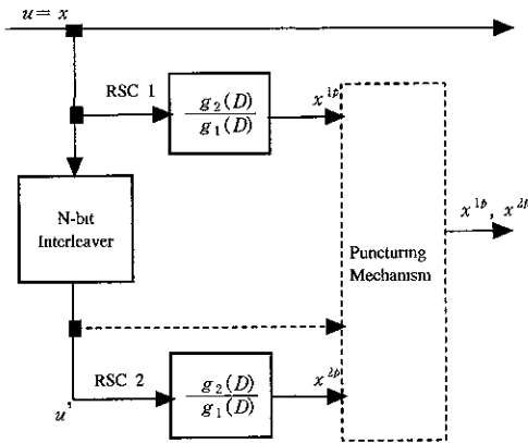
(a) Turbo 인코더 블록도
