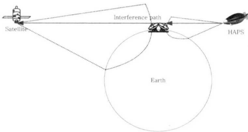
그림 5 Transhorizon path 모델
