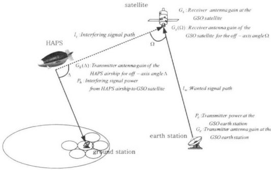
그림 3 HAPS 비행선으로부터 GSO 위성으로의 간섭모델
