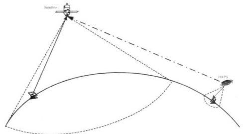
그림 6 Backlobe path 모델
