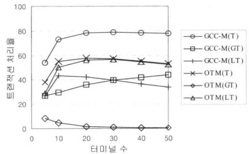
그림 5. 균일 환경에서 터미널 수 변화에 따른 트랜잭션 처리율
