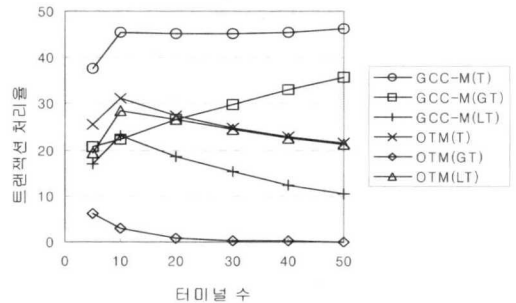
그림 3. 높은 충돌 환경에서 터미널 수 변화에 따른 트랜잭션 처리율
