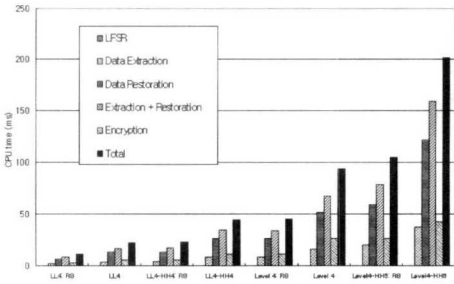
그림 11. 암호화 과정에서 단계별 시간소모
