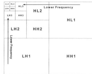
그림 7. 2D DWT 결과의 부대역
