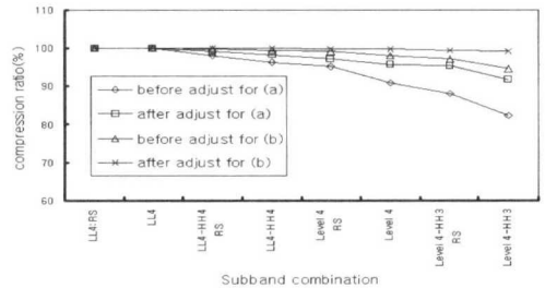
그림 10. 허프만 코드 조정에 의한 압축율 복원
