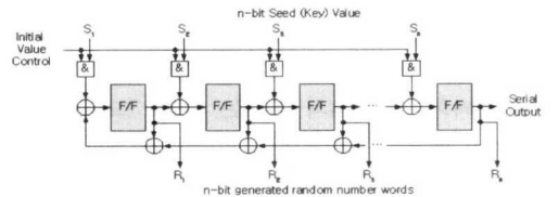
그림 7. 무작위 패턴 생성을 위한 LFSR
