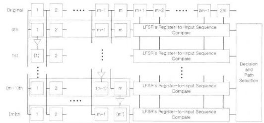
그림 2. 순차 예측기 구조
