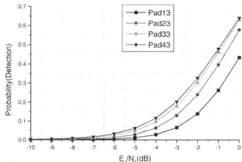
그림 6. E_c/N_0 와 결정 요소 \gamma_1 과 \gamma_2 의 변화에 따른 검출 성능
