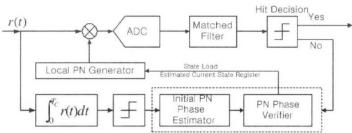
그림 1. 순차 예측 방법을 이용한 포착 시스템
