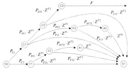
그림 5. 순차 예측 포착을 위한 신호 흐름도
