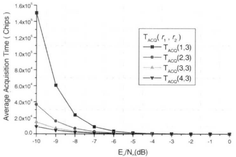
그림 8. \gamma_2 가 3인 경우 E_c/N_0 와 결정 요소 \gamma_1 의 변화에 따른 평균 포착 시간
