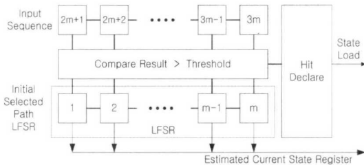
그림 3. 확인 모드에서 사용되는 비교기 구조
