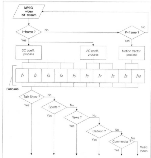
그림 14. 작업 흐름도
