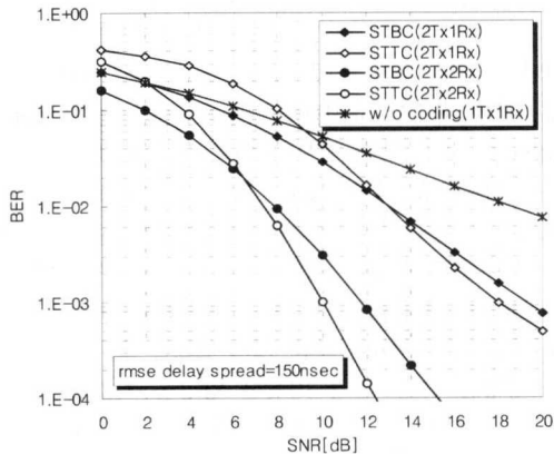
그림 14. BER 성능(rms delay spread=150nsec)
