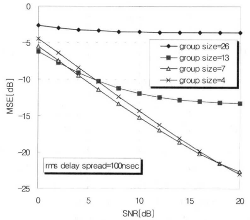
그림 6. MSE 성능(rms delay spread=100nsec)
