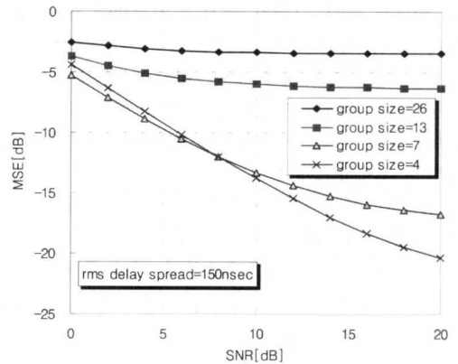
그림 7. MSE 성능(rms delay spread=150nsec)
