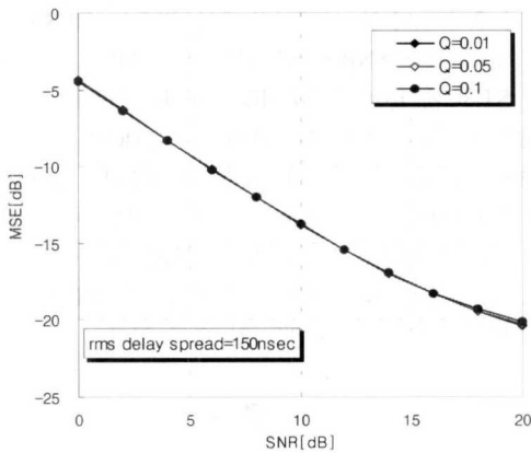
그림 10. MSE 성능(rms delay spread=150nsec)
