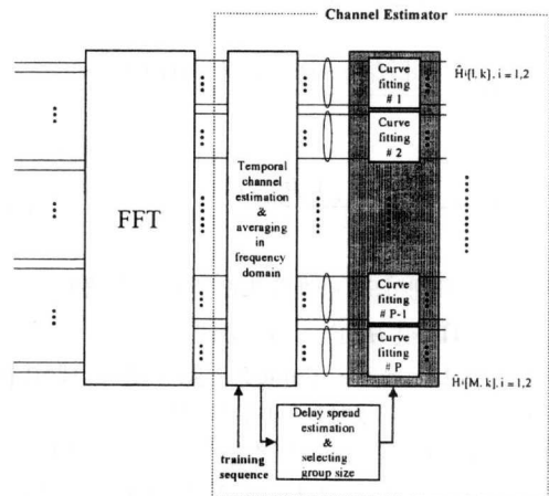
그림 3. curve fitting을 이용한 채널 추정기법
