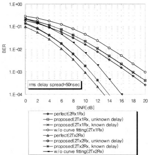
그림 11. STBC의 BER 성능(rms delay spread=50nsec)
