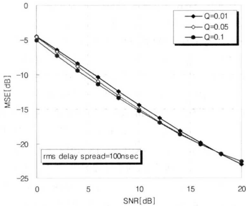
그림 9. MSE 성능(rms delay spread=100nsec)
