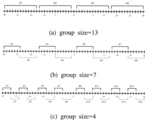
그림 4. IEEE802.11a 시스템에 curve fitting을 위한 그룹의 형성
