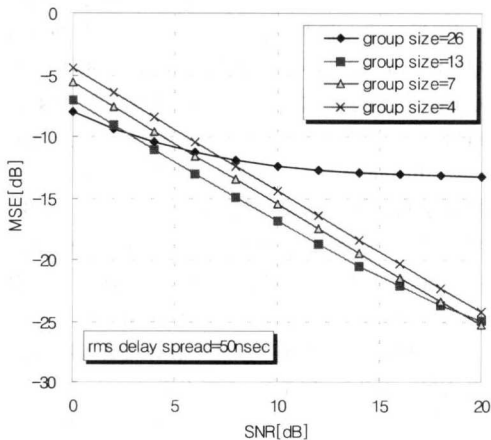
그림 5. MSE 성능(rms delay spread=50nsec)
