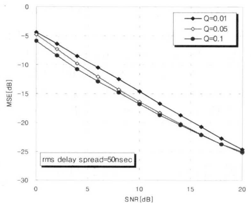
그림 8. MSE 성능(rms delay spread=50nsec)
