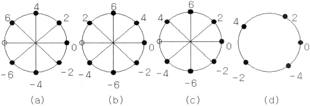
그림 5. MP/CDMA 위상할당 방식
