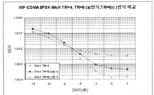
그림 9. MP/CDMA clipping 레벨과 보호위상에 따른 성능 비교(64채널)
