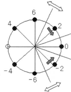
그림 6. clipping 레벨 차를 고려한 위상할당 방안
