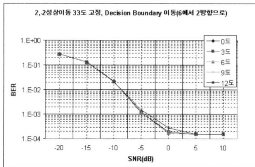
그림 11. Decision Boundary 변화에 따른 성능 비교
