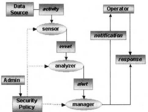
그림 3. IETF IDWG의 Model
