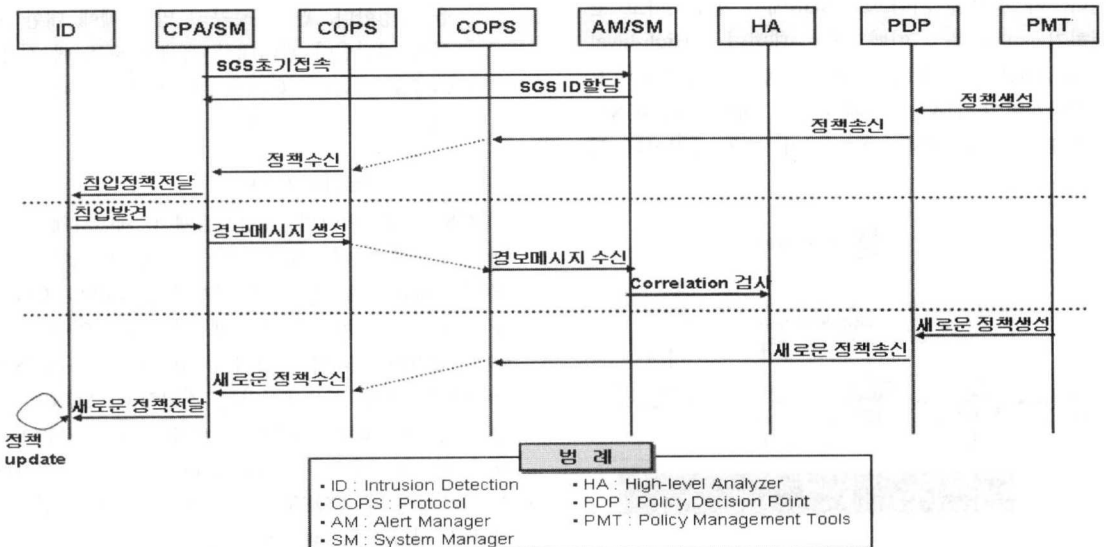
그림 9. 정책기반 보안프레임워크의 흐름도
