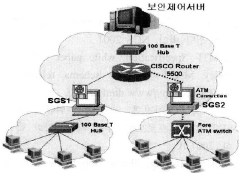
그림 10. 테스트베드 프레임워크 구성
