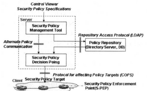
그림 4. IETF의 정책기반 망 관리구조
