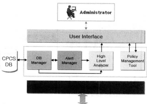
그림 7. 보안제어서버의 기능 블록도
