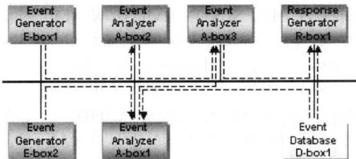
그림 2. CIDF Model
