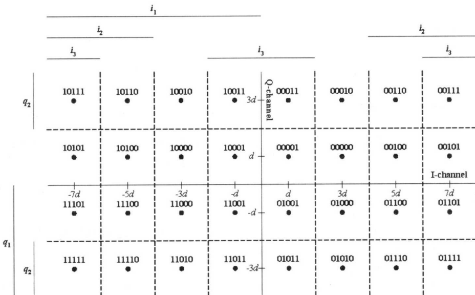
그림 2. 32(8×4)-QAM의 신호 배치도
