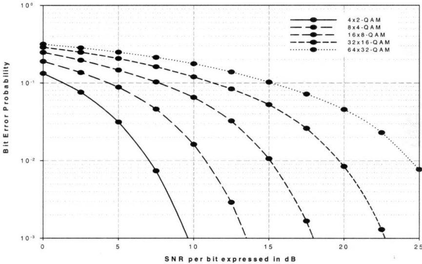
그림 3. AWGN 채널에서 rectangular QAM 신호의 평균 BER
