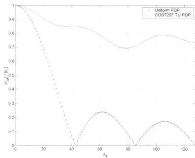
그림 2. N_c = 256, L = 5 인 채널에서 OFDM 부채널 상관특성
