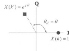
그림 4. 상관도가 가장 낮은 두 부채널로 전송되는 심볼의 성상도 Fig. 4. Constellation of symbol transmitted to the sub channel of the least correlation property
