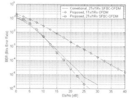
그림 8. 주파수 다이버시티 기법을 적용한 2Tx/1Rx SFBC-OFDM 시스템의 성능 Fig. 8. Performance of 2Tx/1Rx OFDM systems with Frequency diversity scheme
