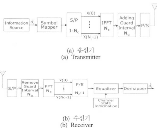
그림 1. OFDM 시스템 Fig 1. OFDM System
