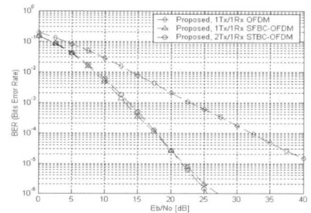
그림 9. 주파수 다이버시티 기법을 적용한 2Tx/1Rx STBC-OFDM과 2Tx/1Rx SFBC-OFDM 시스템의 성능 비교 Fig. 9. Performance comparison of 2Tx/1Rx SFBC-OFDM system with 2Tx/1Rx STBC-OFDM system with frequency diversity scheme
