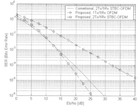
그림 7. 주파수 다이버시티 기법을 적용한 2Tx/1Rx STBC-OFDM 시스템의 성능 Fig. 7. Performance of 2Tx/1Rx OFDM systems with Frequency diversity scheme
