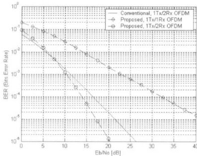
그림 6. 주파수 다이버시티 기법을 적용한 1Tx/2Rx OFDM 시스템의 성능 Fig. 6. Performance of 1Tx/2Rx OFDM system with Frequency diversity scheme
