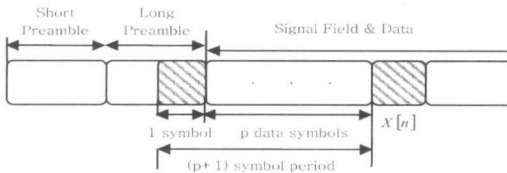
그림 8. SFBC 기법을 위한 MIMO-OFDM 시스템의 프레임 구조 Fig. 8. The frame structure of the MIMO-OFDM system for the SFBC scheme
