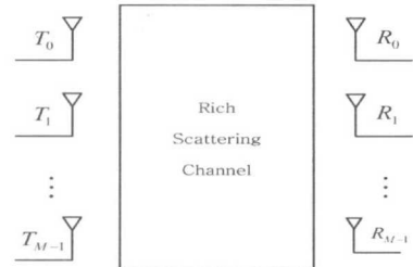
그림 2. MIMO-OFDM 시스템의 채널 구조 Fig. 2. The channel structure of the MIMO-OFDM system
