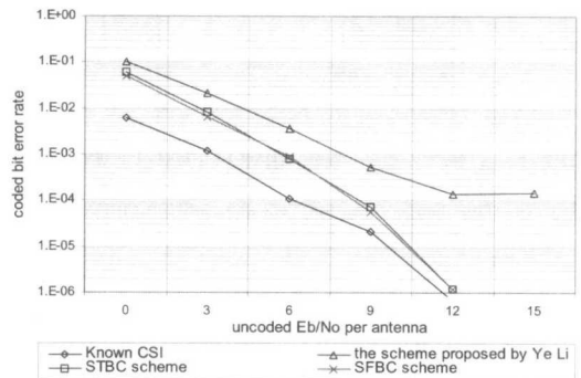
그림 9. 50ns RMS 지연 확산 페이딩 채널 환경에서 24Mbps의 전송률을 가지는 MIMO-OFDM 시스템의 각 채널 추정 기법에 따른 비트 에러 성능 곡선 Fig. 9. The bit error performance of the MIMO-OFDM system with 24Mbps data rate in 50ns RMS delay spread fading channel
