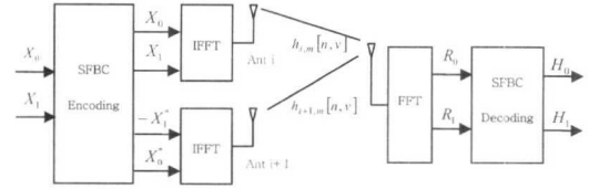
그림 7. SFBC 기법이 적용된 MIMO-OFDM시스템의 송수신 구조 Fig. 7. The structure of the transmitter and receiver of the MIMO-OFDM system for the SFBC scheme
