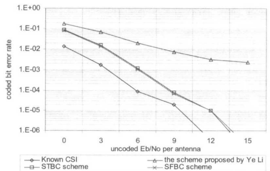
그림 10. 50ns RMS 지연 확산 페이딩 채널 환경에서 48Mbps의 전송률을 가지는 MIMO-OFDM 시스템의 각 채널 추정 기법에 따른 비트 에러 성능 곡선 Fig. 10. The bit error performance of the MIMO-OFDM system with 48Mbps data rate in 50ns RMS delay spread fading channel
