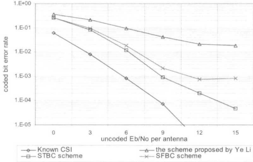
그림 14. 150ns RMS 지연 확산 페이딩 채널 환경에서 48Mbps의 전송률을 가지는 MIMO-OFDM 시스템의 각 채널 추정 기법에 따른 비트 에러 성능 곡선 Fig. 14. The bit error performance of the MIMO-OFDM system with 48Mbps data rate in 150ns RMS delay spread fading channel
