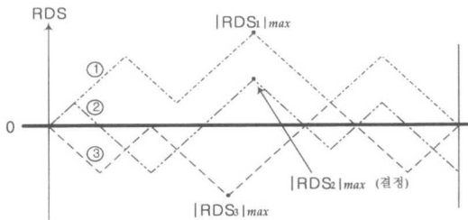
그림 4. MPRDS 방법을 적용한 예
