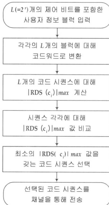
그림 3. 제안된 MPRDS 방법에 대한 순서도
