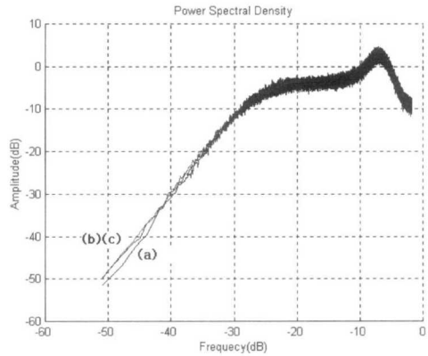
(1) 2비트의 제어 비트를 삽입한 경우
