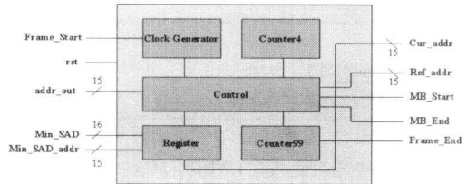
그림 9. 제어 블록
