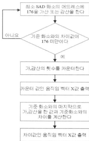
그림 7. 움직임 벡터 제너레이터 블록 동작 순서
