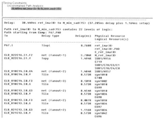
그림 18. 시스템 타이밍 분석
