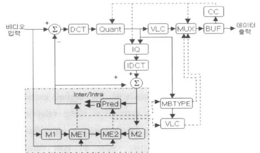
그림 1. H.263 엔코더 블록도
