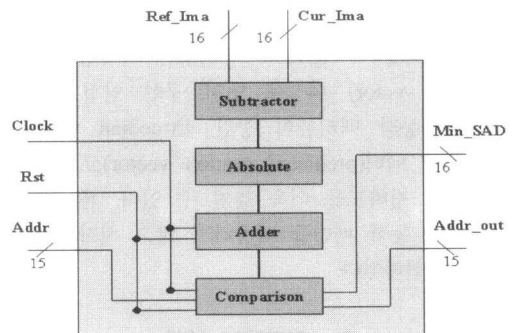
그림 6. SAD 블록
