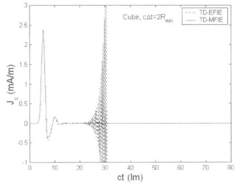
그림 5. 정육면 도체 윗면 중앙의 x 방향 전류의 지연응답. c\Delta t = 2R_{\min} .
