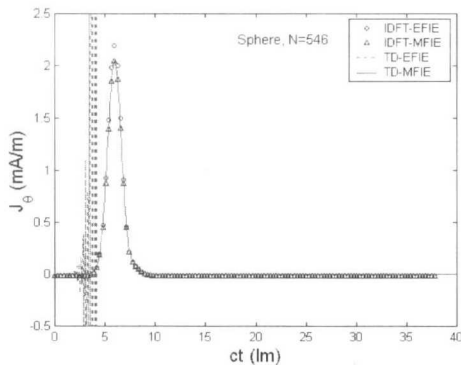
그림 9. 도체구 상의 \theta=90^\circ , \phi=13^\circ 에서 \theta 방향 전류의 지연 응답.
