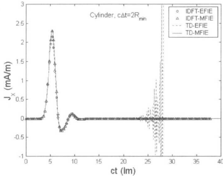
그림 11. 원통 도체 윗면의 x 방향 전류의 지연응답. c\Delta t = 2R_{min} .
