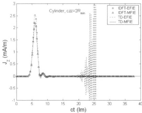
그림 12. 원통 도체 옆면의 z 방향 전류의 지연응답. c\Delta t = 2R_{min} .
