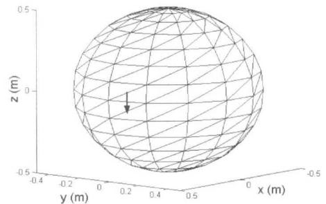
그림 6. 도체구의 삼각형 분할.
