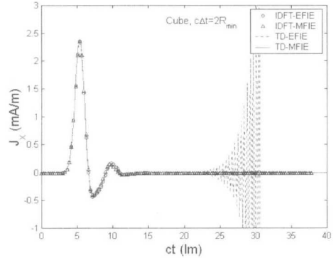
그림 4. 정육면 도체 윗면 중앙의 x 방향 전류의 지연응답. c\Delta t = 2R_{\min} .
