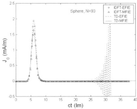
그림 7. 도체구 상의 \theta=90^\circ , \phi=30^\circ 에서 \theta 방향 전류의 지연 응답.
