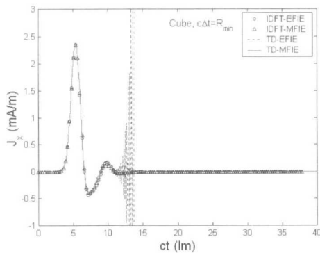
그림 3. 정육면 도체 윗면 중앙의 x 방향 전류의 지연응답. c\Delta t = R_{\min} .
