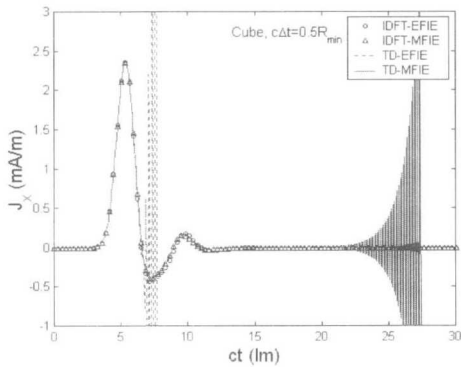
그림 2. 정육면 도체 윗면 중앙의 x 방향 전류의 지연응답. c\Delta t = 0.5R_{\min} .
