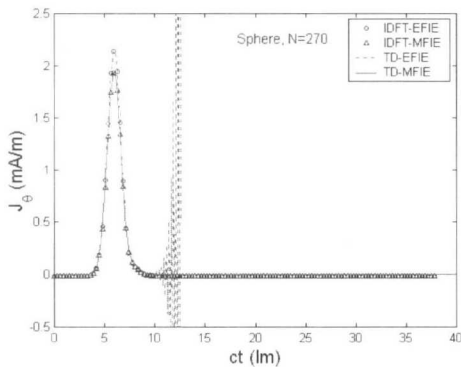
그림 8. 도체구 상의 \theta=90^\circ , \phi=18^\circ 에서 \theta 방향 전류의 지연 응답.
