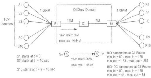
그림 9. AS 플로간의 공평성 보장에 대한 시뮬레이션 모델
