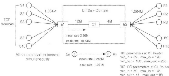
그림 4. RIO-DC 변수 설정 방안에 대한 시뮬레이션 모델
