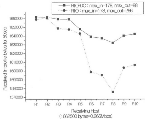
그림 10. 그림 9에서 각 호스트의 50초간 수신 In-byte 수
