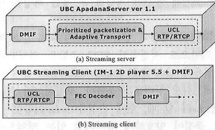
그림 4. 구현 소프트웨어 아키텍처.
