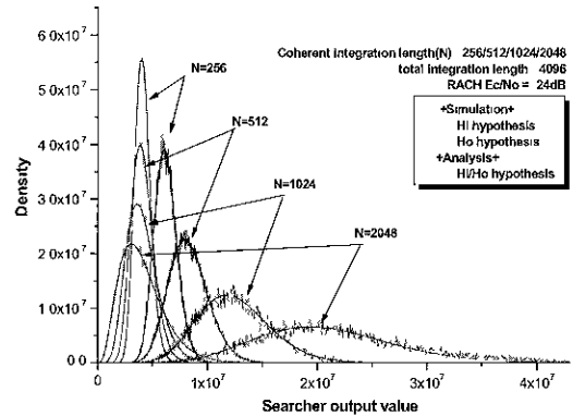
그림 7 동기 누적 길이에 따른 H_1, H_0 의 확률 밀도 분포
