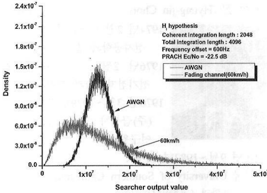
그림 13. 채널 환경에 따른 H_1 가설의 확률 밀도 분포 (AWGN vs. fading(60km/h))
