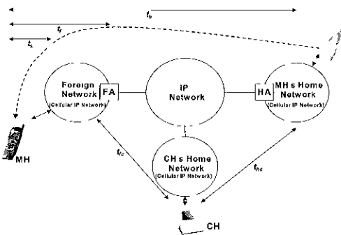
그림 5 핸드오프 지연시간 분석을 위한 네트워크 모델
