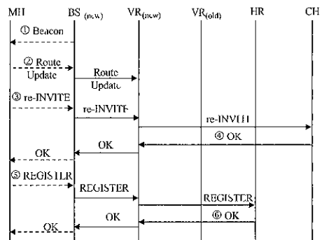
그림 4 SIP/CIP의 메시지 플로우
