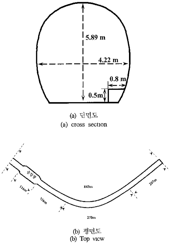
그림 5 터널의 단면도와 평면도 Fig 5 Cross section and top view of the tunnel
