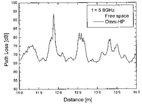
(b) 무지향성 수평편파 안테나 (b) Omnidirectional-HP antenna
