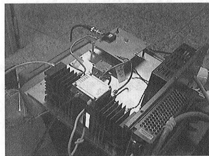
(a) 송신기 시스템 (a) Transmitter system
