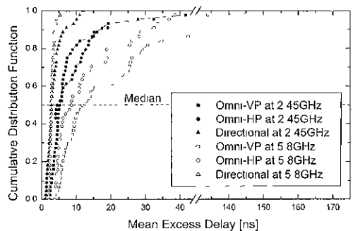
그림 11 평균초과지연의 누적분포함수 Fig 11 CDF of mean excess delay
