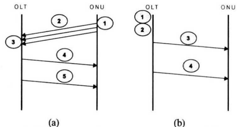
그림 4. Automatic Protection Switching 절차 (a)ONU 사고 감지 (b)OLT 사고 감지
