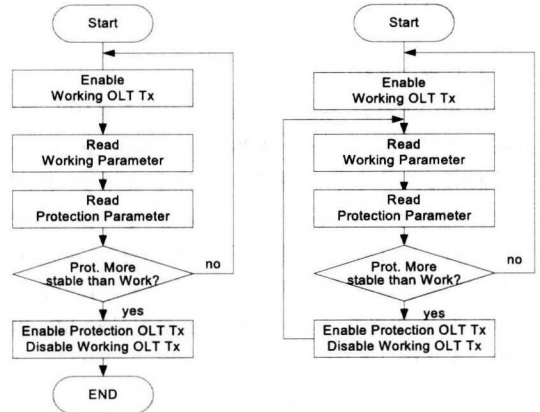
그림 6. OLT 제어용 프로세서의 동작 순서도
