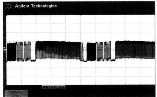
그림 7. 정상 동작 시 OLT에서의 프레임 수신
