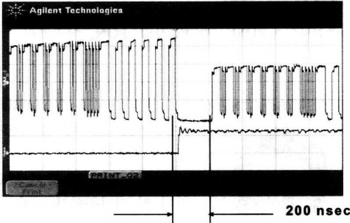
그림 8. 프리앰블 에러 발생시의 OLT 시스템 절체 (위: ONU에서 수신한 OLT 전송신호, 아래: 에러 검출신호)
