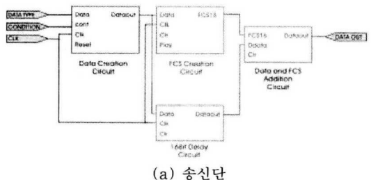
(a) 송신단
