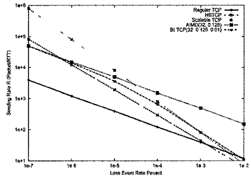
그림 1 TCP 및 High-speed TCP 프로토콜의 응답 함수[7]
