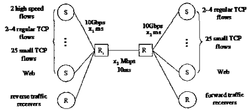
그림 3 시뮬레이션을 위한 망 구성
