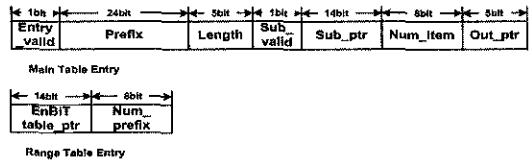
그림 9 엔트리 구조
