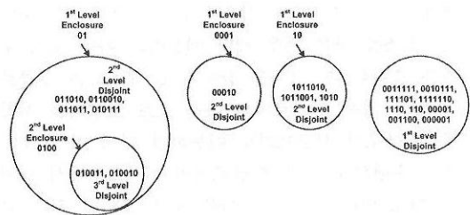
그림 4. 프리픽스 분류
