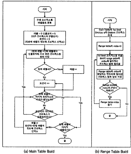
그림 6 제안하는 구조의 빌드 플로차트
