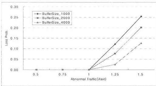
그림 11. 버퍼 크기에 따른 정보 손실
