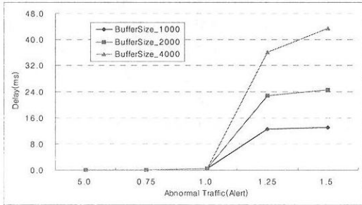
그림 10. 버퍼 크기에 따른 정보 지연
