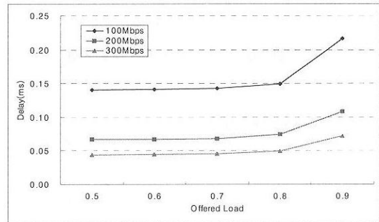
그림 9. 기가비트 스위치를 이용한 정보 지연
