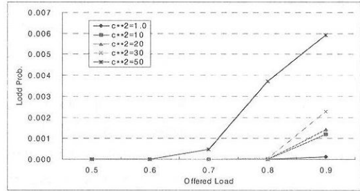
그림 13. 버스티니스 정도에 따른 정보 전송 손실
