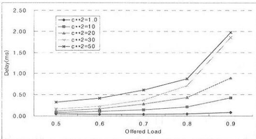
그림 12. 버스티니스 정도에 따른 정보 전송 지연
