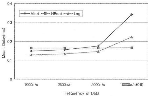
그림 17. 데이터 생성빈도에 따른 지연
